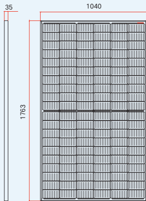
正视图
