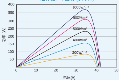
组件的P-V曲线 (370W)
