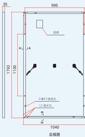
后视图
