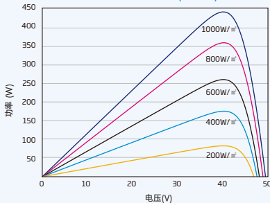
组件的P-V曲线 (445W)
