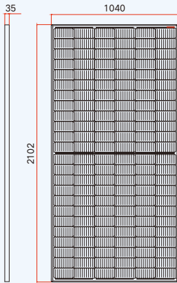
正视图
