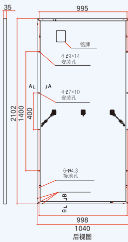
后视图
