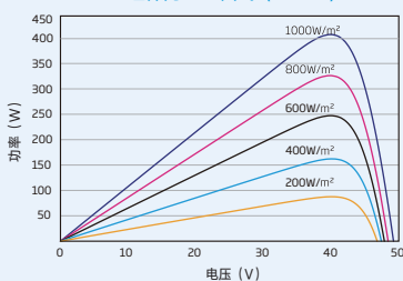
组件的P-V曲线(405W)
