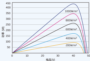
组件的P-V曲线(445W)
