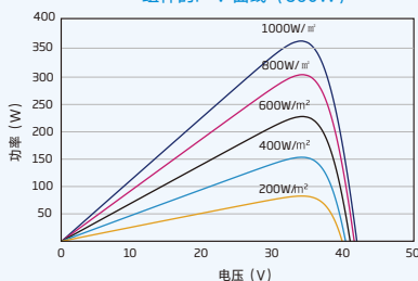
组件的P-V曲线(360W)
