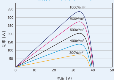
组件的P-V曲线(335W)
