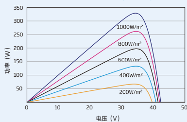
组件的P-V 曲线 (330W)
