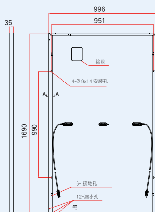
后视图
