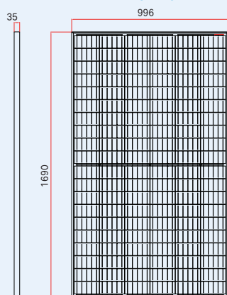
前视图
