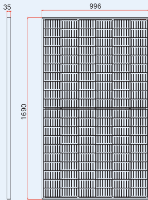
正视图
