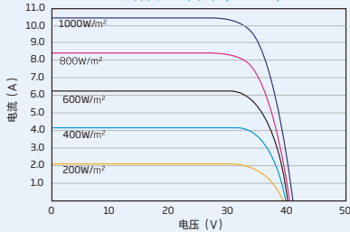
组件的I-V 曲线 (335W)
