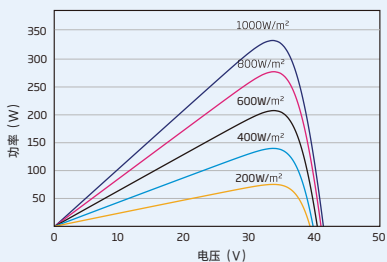
组件的P-V 曲线 (335W)
