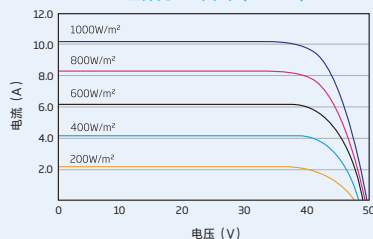
组件的I-V 曲线 (390W)
