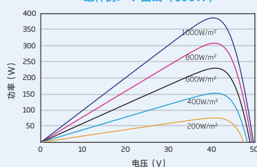
组件的P-V 曲线 (390W)
