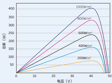
组件的P-V曲线(405W)
