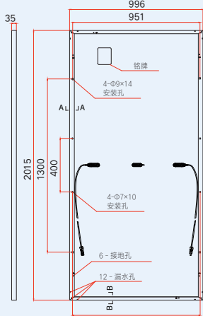
后视图
