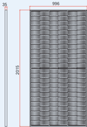
正视图
