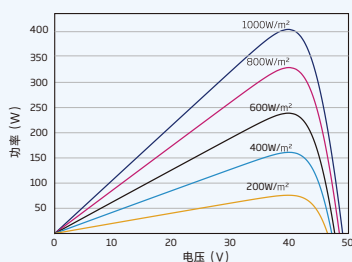
组件的P-V 曲线 (405W)
