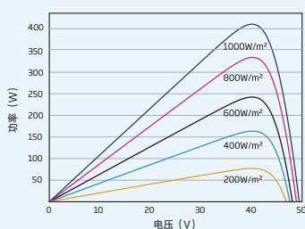
组件的P-V 曲线 (410W)
