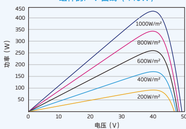
组件的P-V曲线(440W)
