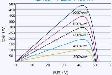
组件的P-V 曲线 (490W)
