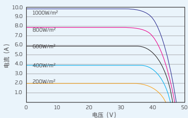
组件的I-V曲线 (365W)
