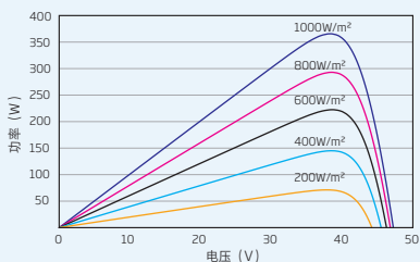
组件的P-V曲线 (365W)
