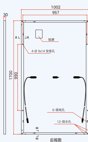
后视图
