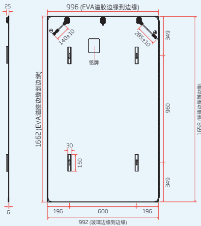
后视图 (竖装)
