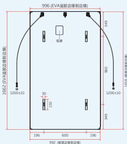
后视图 (横装)
