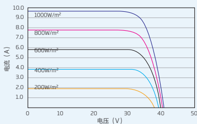
组件的I-V曲线 (305W)
