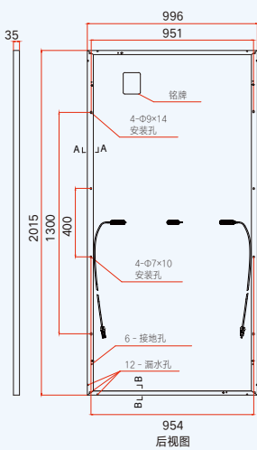
后视图
