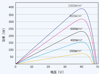
组件的P-V 曲线 (395W)
