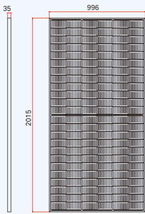
正视图
