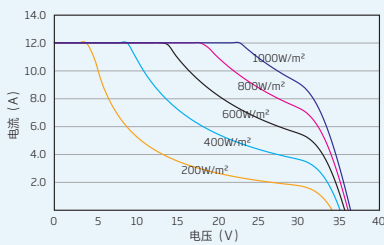
组件的I-V曲线 (275W)
