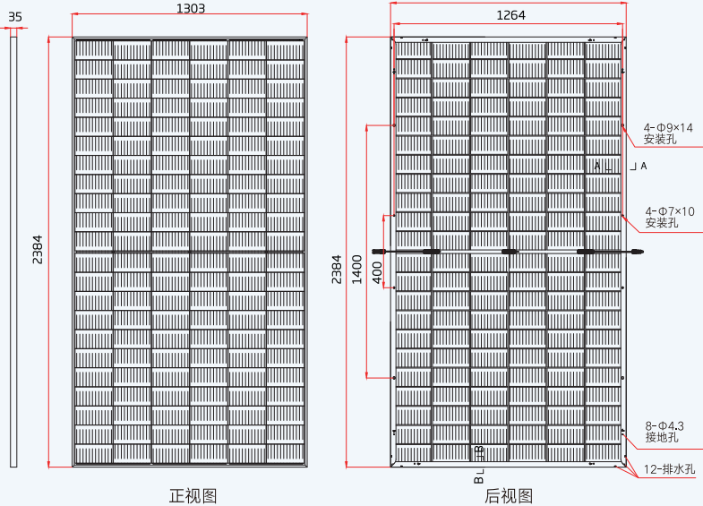
组件尺寸(mm)
