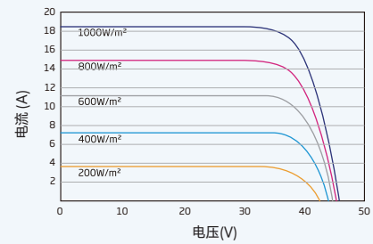
组件的P-V曲线(645W)
