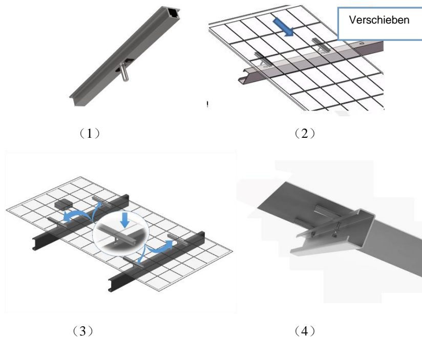
Abbildung 1. Mit Gecko Grip installiertes PV-Modul
