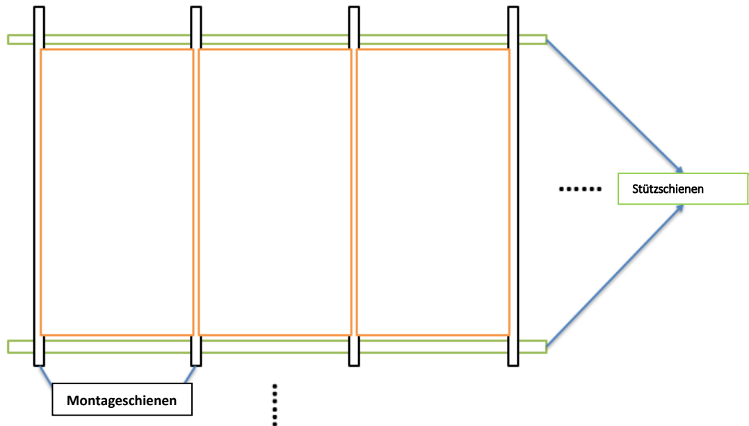
Abbildung 3: Modulzeichnung und Installationskizze
