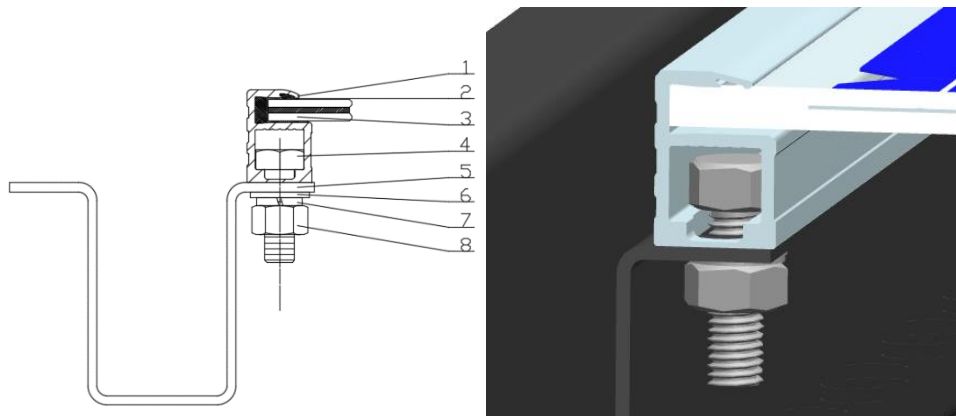
Abbildung 2 Montage mit Rahmen
