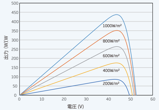
PVモジュール (440W) P-V曲線
