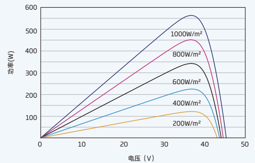
组件的P-V曲线 (565W)
