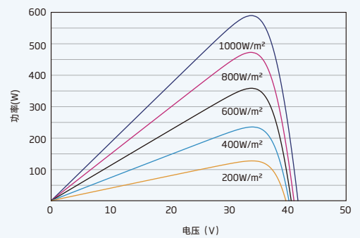
组件的P-V曲线 (600W)
