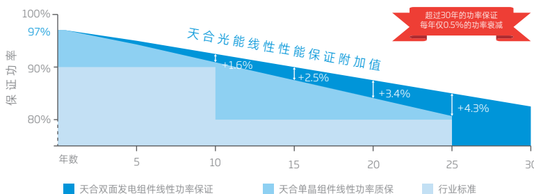
双面发电组件线性功率保证
