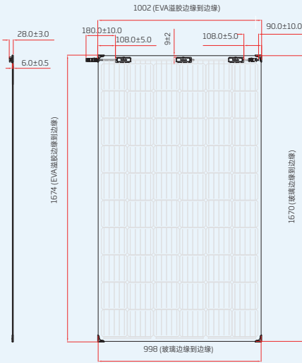
后视图 (竖装)
