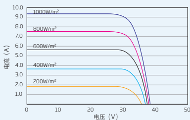
组件的I-V曲线 (280W)
