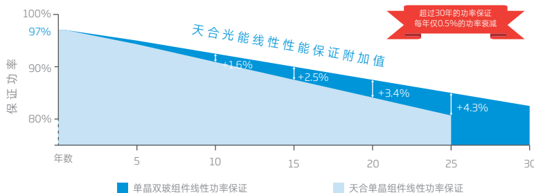
单晶双玻组件线性功率保证
