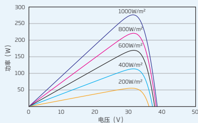
组件的P-V曲线 (280W)
