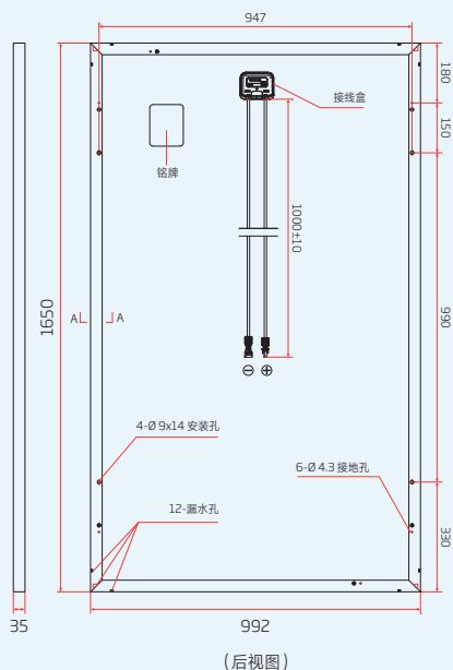
组件尺寸 (mm)
