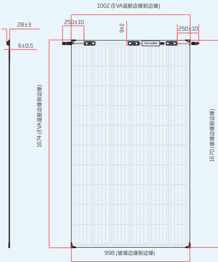
后视图 (竖装)
