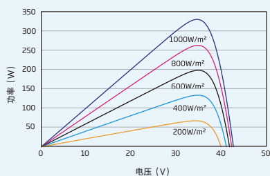
组件的P-V曲线(335W)
