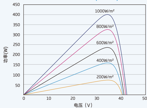
组件的P-V曲线(400W)
