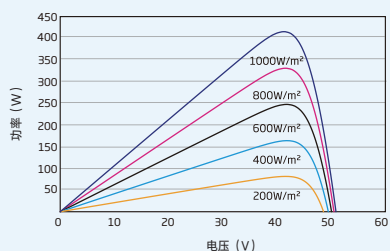
组件的P-V曲线(405W)
