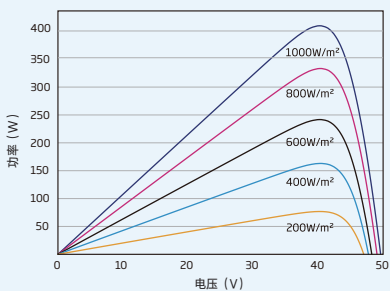
组件的P-V曲线(410W)
