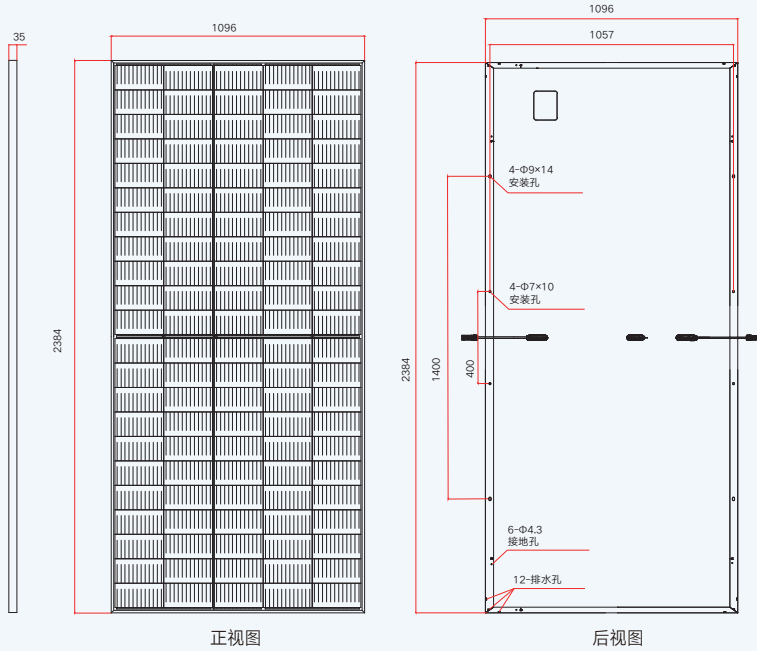
组件尺寸(mm)
