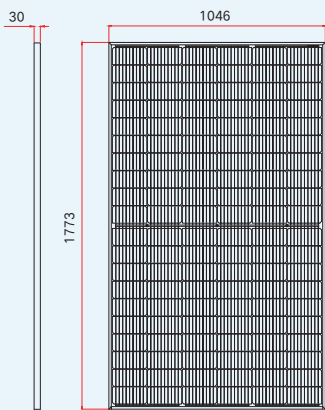
前视图
