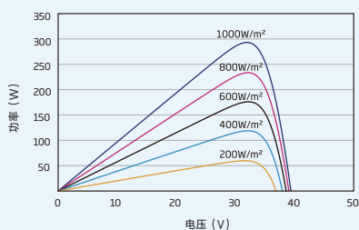
组件的P-V曲线(295W)
