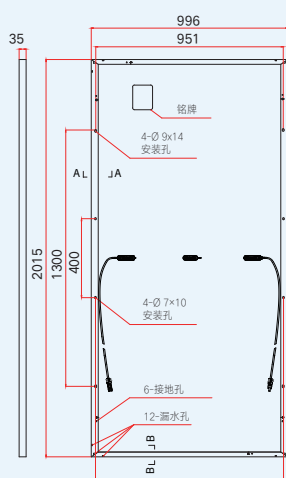
后视图
