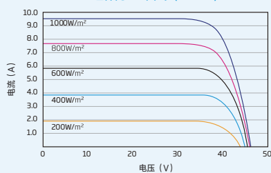
组件的I-V 曲线 (345W)
