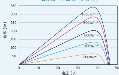
组件的P-V 曲线 (345W)
