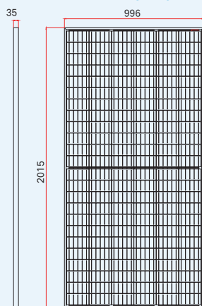
正视图
