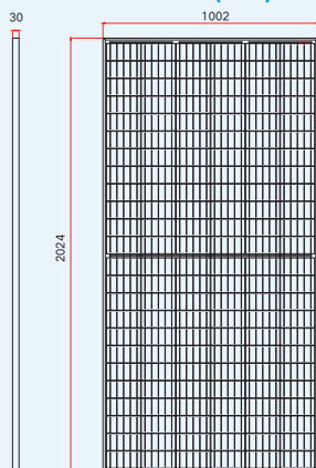
前视图
