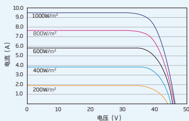
组件的I-V 曲线 (345W)
