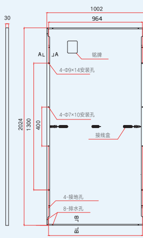
后视图
