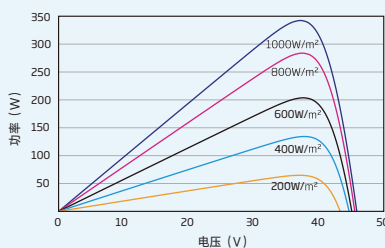
组件的P-V 曲线 (345W)
