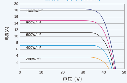
组件的P-V曲线 (650W)
