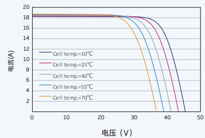
组件的I-V曲线 (650W)
