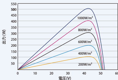
PVモジュール(505 W)のP-V曲線
