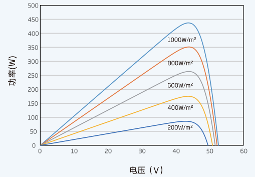
组件的P-V曲线(440W)
