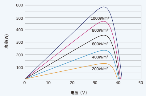
组件的P-V曲线 (595W)
