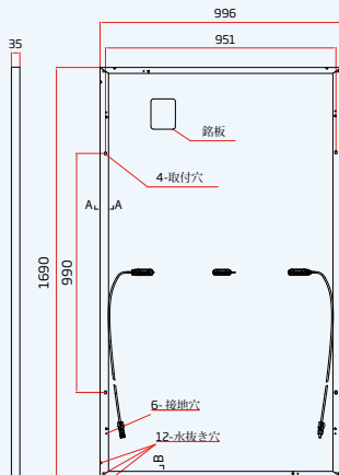
裏面図
