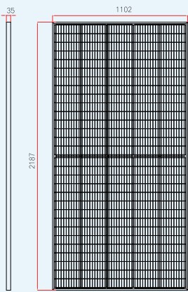
正视图
