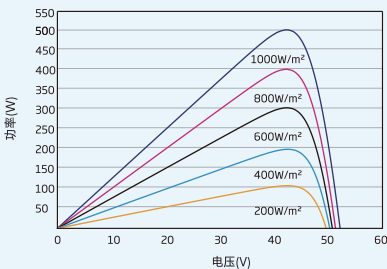
组件的P-V曲线 (500W)
