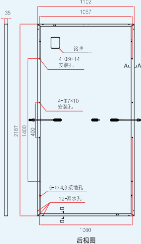
后视图
